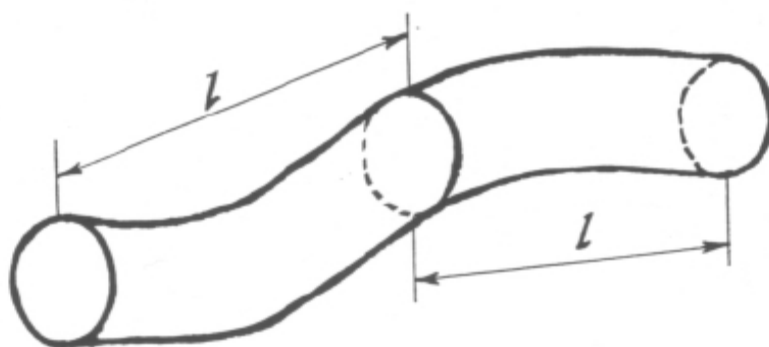
2 iliustracija. Apvaliosios medienos su sudėtinguoju kreivumu ilgio matavimas
