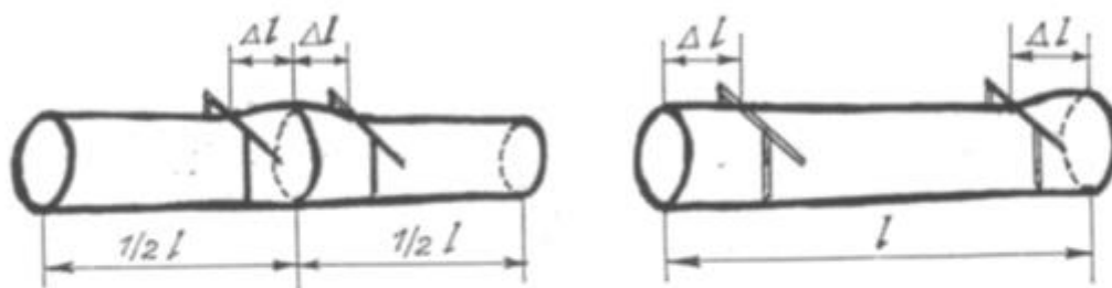
5 iliustracija. Rąstų skersmens matavimas, kai matavimo vietoje yra kliuvinys.
