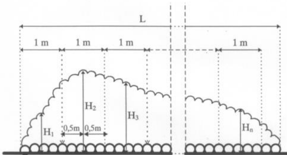
8 iliustracija. Rietuvės aukščio matavimas.
