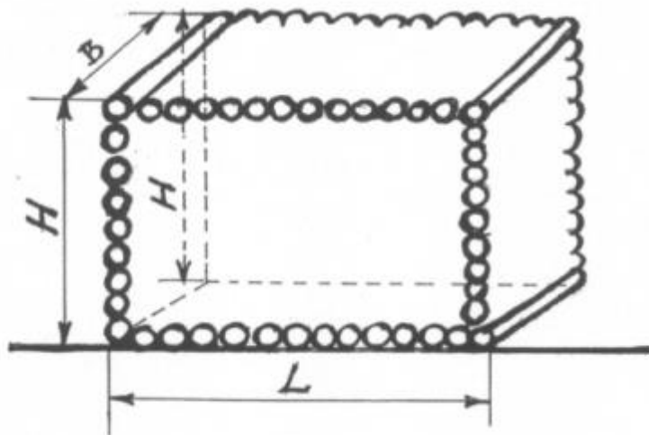
7 iliustracija. Rietuvės matmenų nustatymas.
