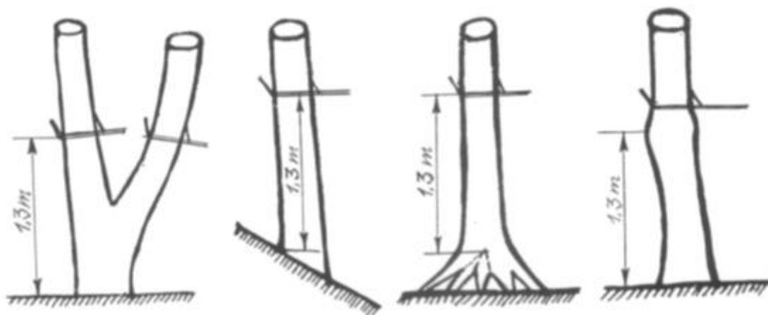
6 iliustracija. Nenukiršto medžio stiebo skersmens matavimas 1,3 m aukštyje.
