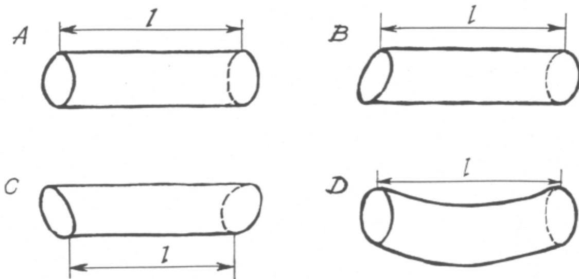
1 iliustracija. Tiesios (A, B, C) ir su paprastuoju kreivumu (D) apvaliosios medienos ilgi matavimas
