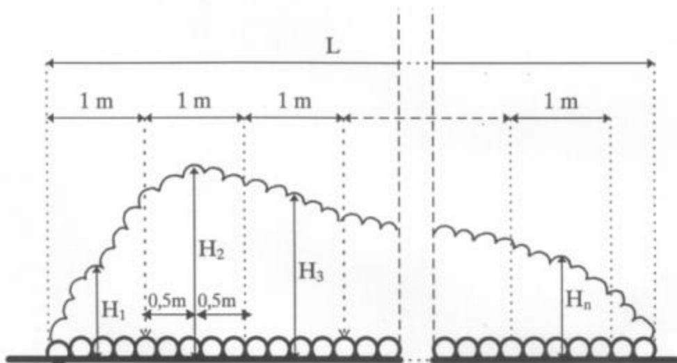
8 iliustracija. Rietuvės aukščio matavimas.
