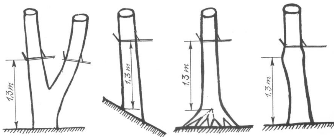
6 iliustracija. Nenukirto medžio stiebo skersmens matavimas 1,3 m aukštyje.
