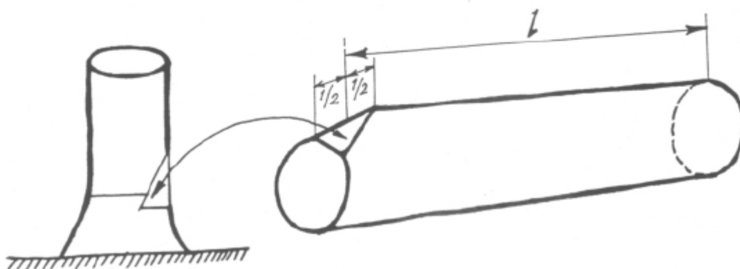
3 iliustracija. Apvaliosios medienos su įpjovimu ilgio matavimas
