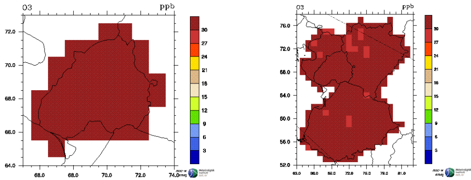
5 paveikslas. O 3 koncentracijos Lietuvoje (kairė) ir kaimyninėse šalyse (dešinė) (duomenų šaltinis: EMEP/MSC-W modeliujama oro koncentracija ir iškritos. Duomenų bazė ( angl. EMEP/MSC-W modelled air concentrations and depositions ). Prieiga internetu: http://www.emep.int/mscw/mscw_ydata.html )
