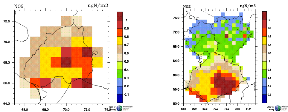
2 paveikslas. \text{NO}_x iškritos Lietuvoje (kairė) ir kaimyninėse šalyse (dešinė) (duomenų šaltinis: EMEP/MSC-W modeliuojama oro koncentracija ir iškritos. Duomenų bazė (angl. EMEP/MSC-W modelled air concentrations and depositions). Prieiga internetu: http://www.emep.int/mscw/mscw_ydata.html )
