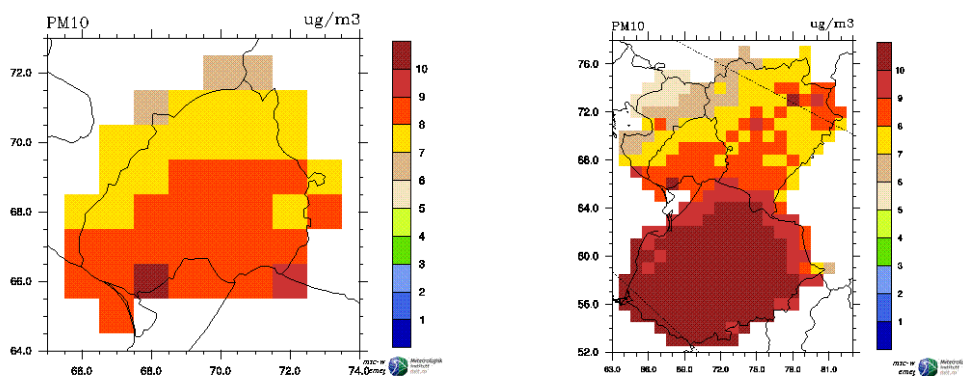
3 paveikslas. \text{KD}_{10} iškritos Lietuvoje (kairė) ir kaimyninėse šalyse (dešinė) (duomenų šaltinis: EMEP/MSC-W modeliuojama oro koncentracija ir iškritos. Duomenų bazė (angl. EMEP/MSC-W modelled air concentrations and depositions). Prieiga internetu: http://www.emep.int/mscw/mscw_ydata.html )
