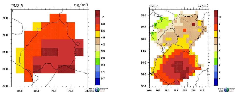
4 paveikslas. KD 2,5 iškritos Lietuvoje (kairė) ir kaimyninėse šalyse (dešinė) (duomenų šaltinis: EMEP/MSW modeliujama oro koncentracija ir iškritos. Duomenų bazė ( angl. EMEP/MSW modelled air concentrations and depositions ). Prieiga internetu: http://www.emep.int/mscw/mscw_ydata.html )
