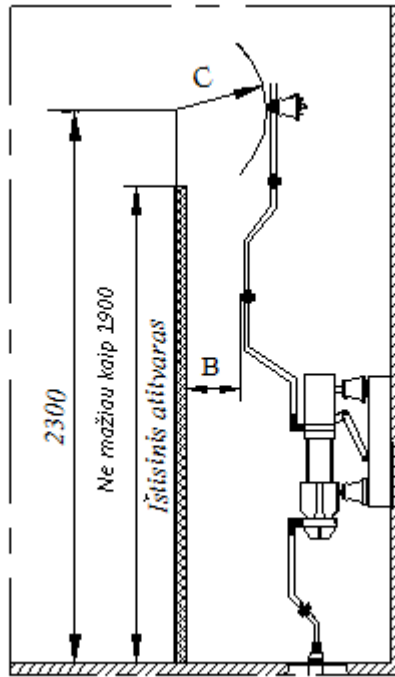
14 paveikslas. Mažiausi atstumai tarp neizoliuotų srovėlaidžių ir išsistinių atitvarų (2 lentelė)
