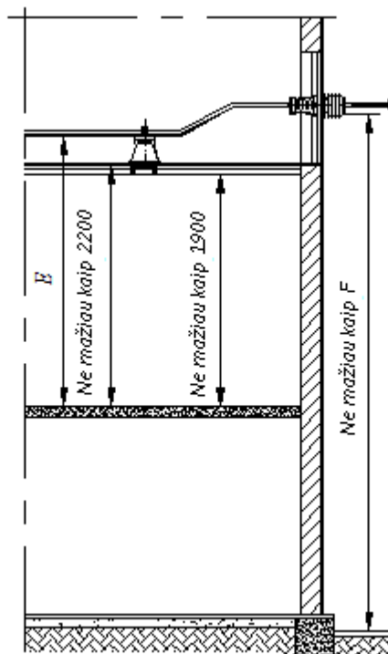
16 paveikslas. Mažiausi atstumai nuo grindų iki neatitvertų srovėlaidžių, iki apatinio izoliatoriaus porceliano krašto ir nuo žemės iki uždarnosios skirstyklos neatitvertų linijinių įvadų iš atvirosios skirstyklos teritorijos, po kuria nėra važiuojamųjų kelių
