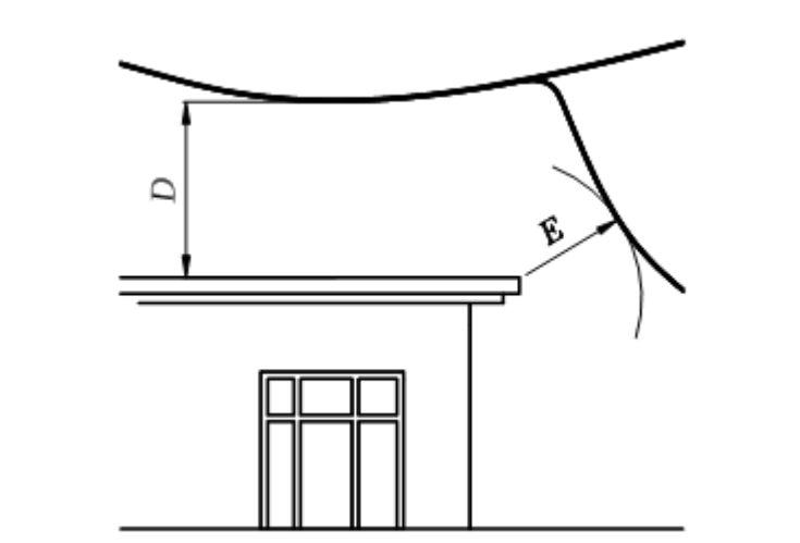
10 paveikslas. Mažiausi atstumai tarp srovėlaidžių ir statinių
